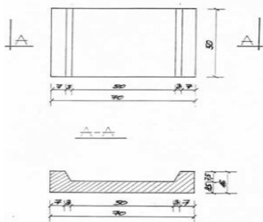
KORYTO ŚCIEKOWE 16 x 50 x 70 TYP HAŁCNÓW
