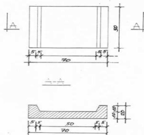
KORYTO ŚCIEKOWE 20 x 50 x 70 TYP HAŁCNÓW
